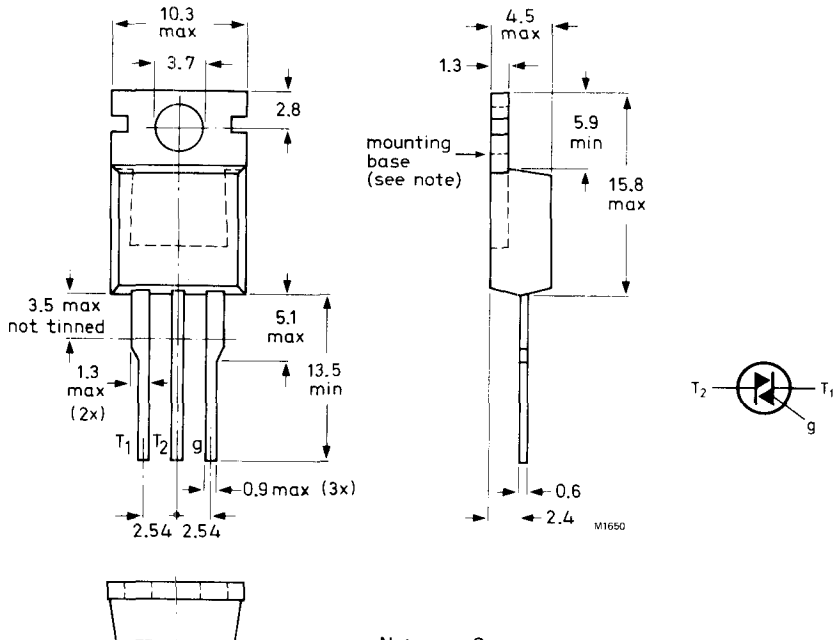
Fig.1 TO-220AB.
