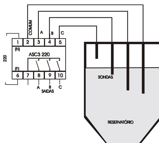
Esquema de ligação
